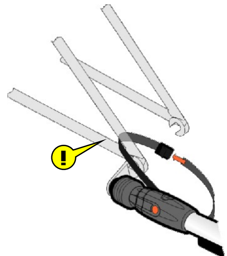
Abb. 5: Sicherheitsfangband um Rahmen legen
